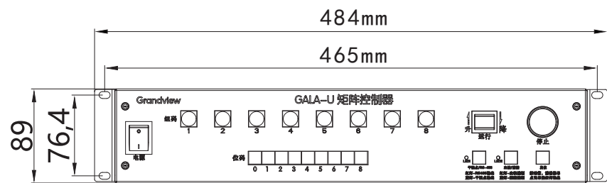
正视图
